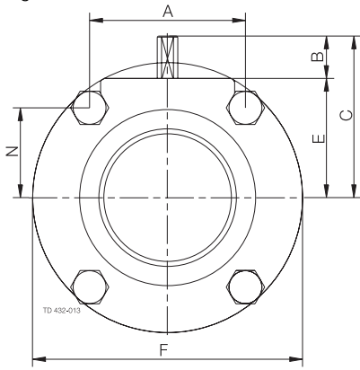
Fig. 1. Dimensions - vanne.
